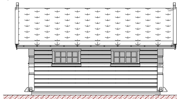
Fasade mot
