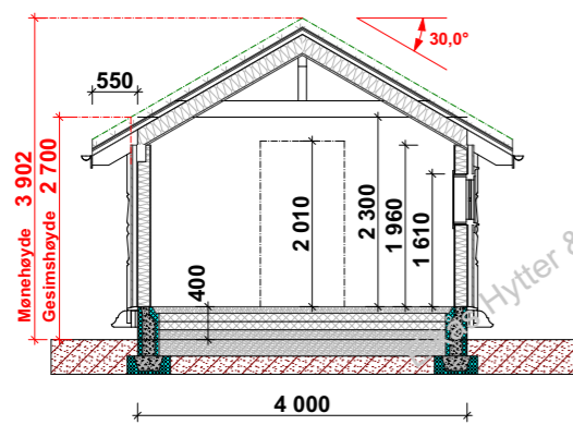
Snitt B-B
