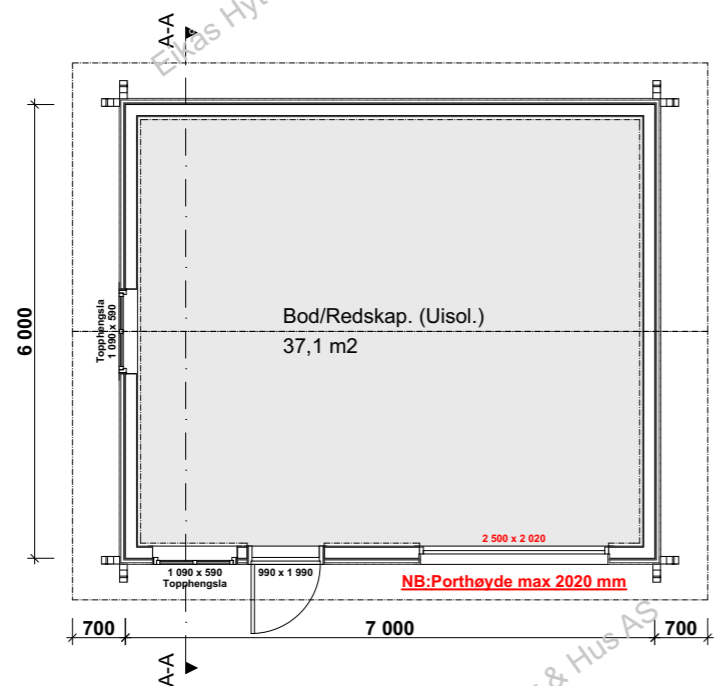
Hovedplan
