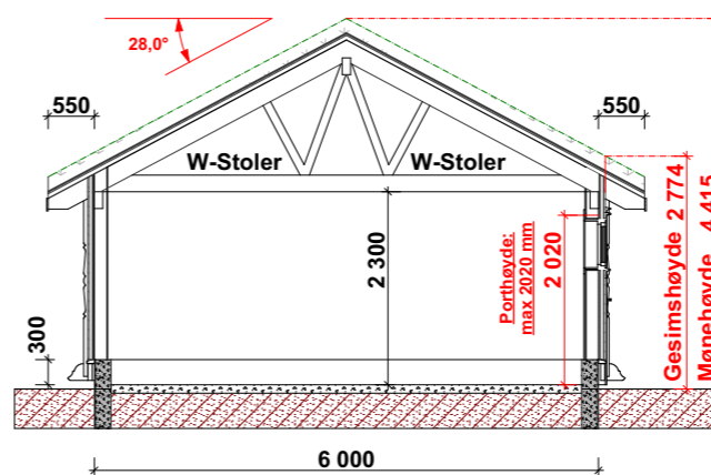
Snitt A-A
