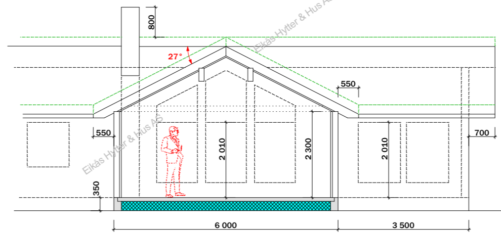
Snitt 2
