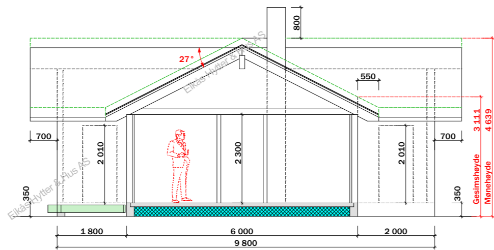
Snitt 1
