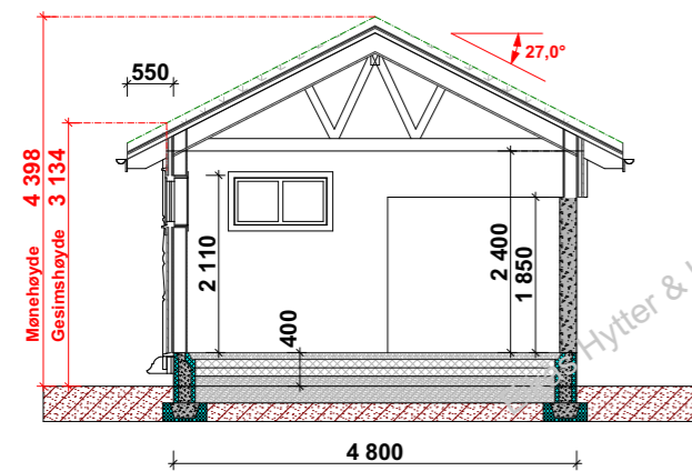
Snitt A-A
