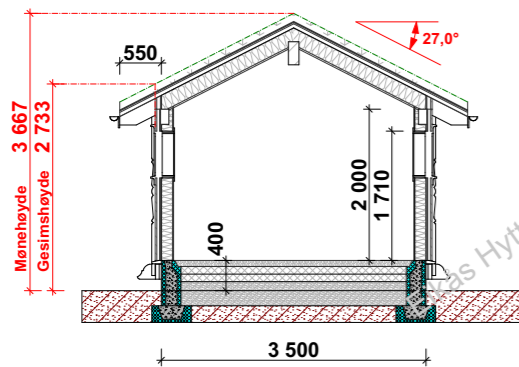
Snitt B-B
