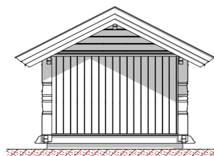
Fasade mot
