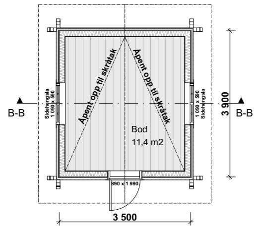
Hovedplan
