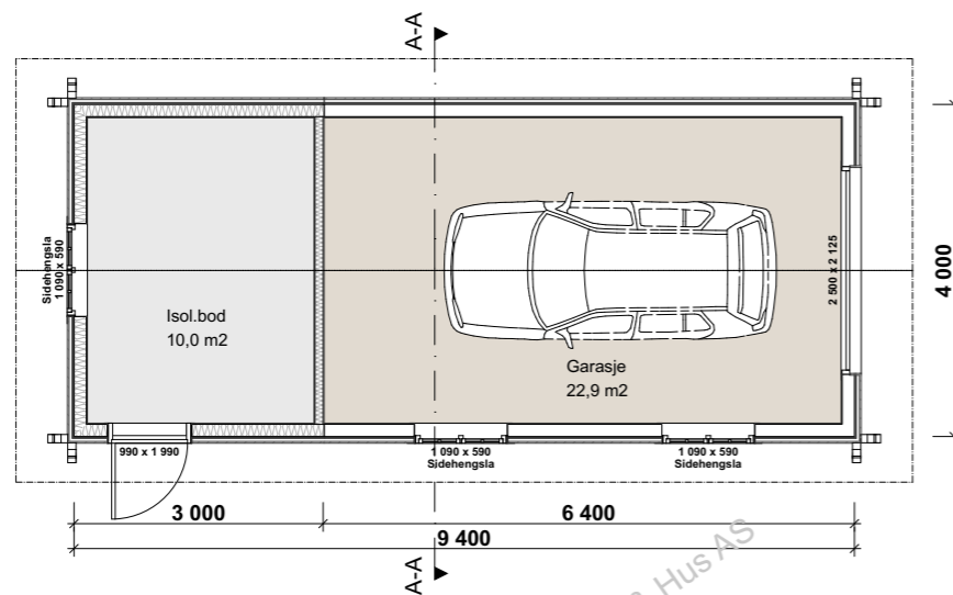
Hovedplan
