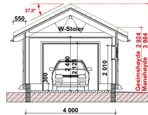
Snitt A-A
