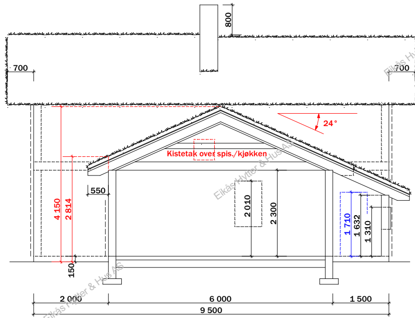
Snitt 2
