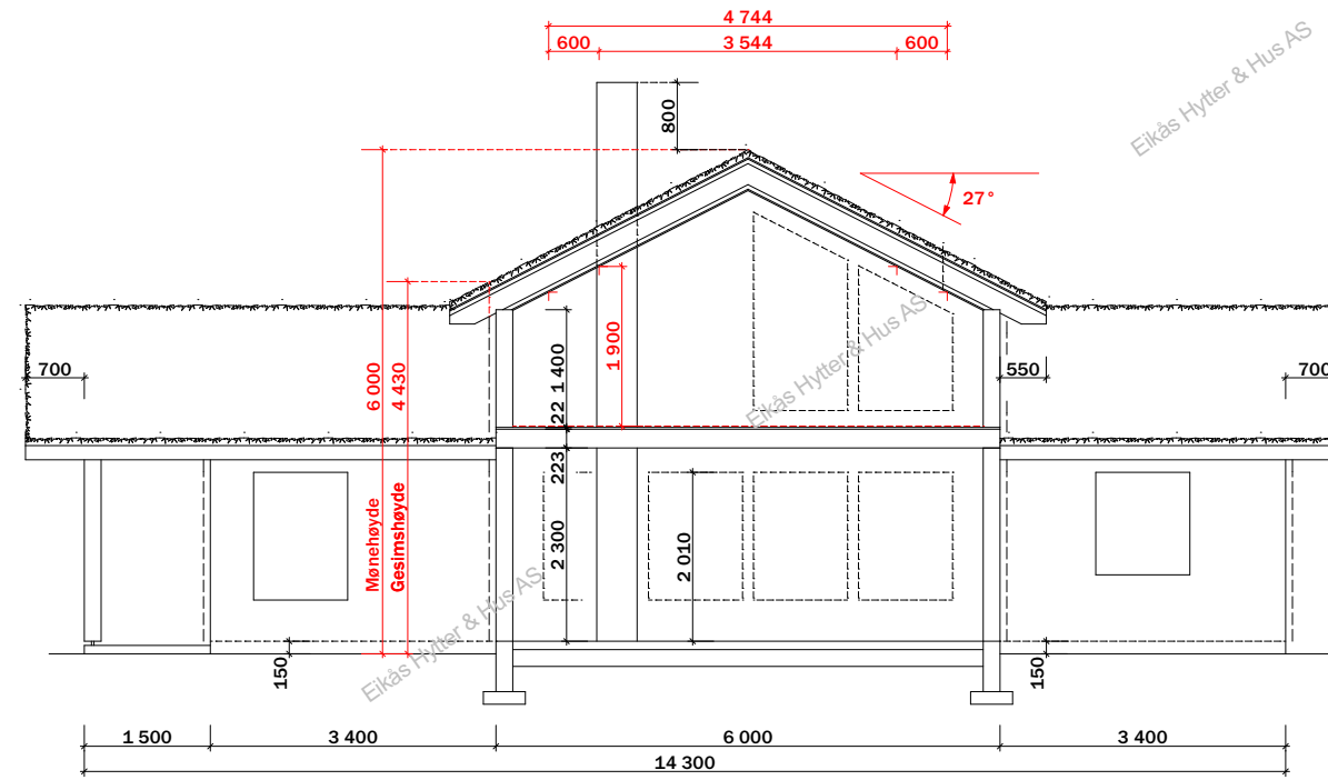
Snitt 1
