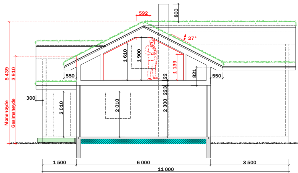
Snitt 2
