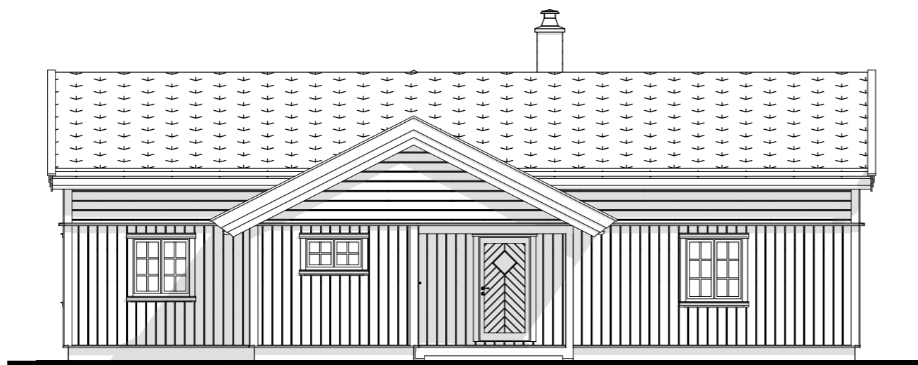
Fasade mot
