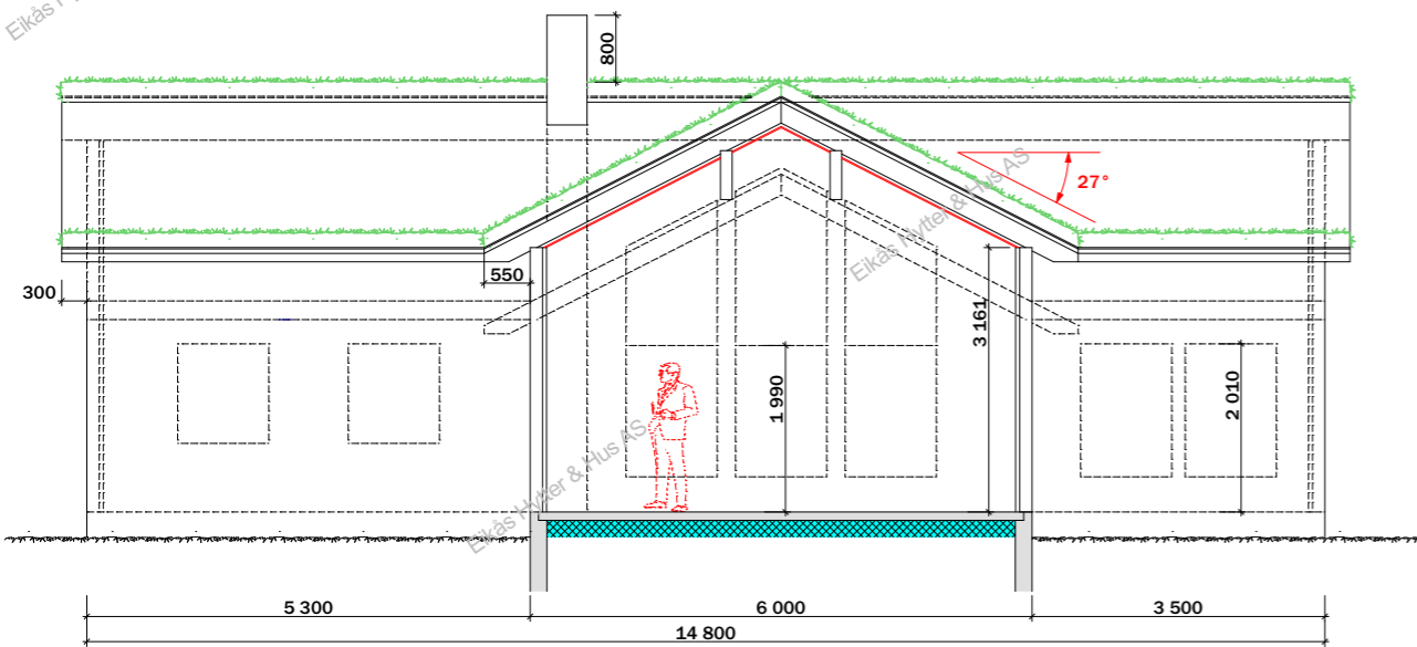
Snitt 1
