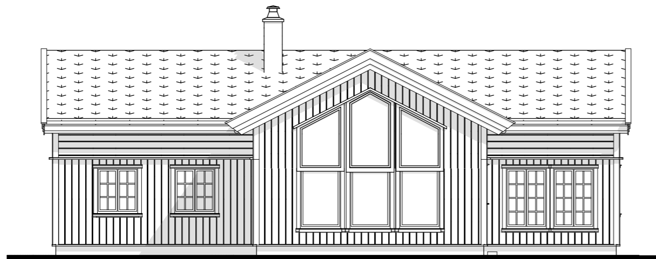
Fasade mot
