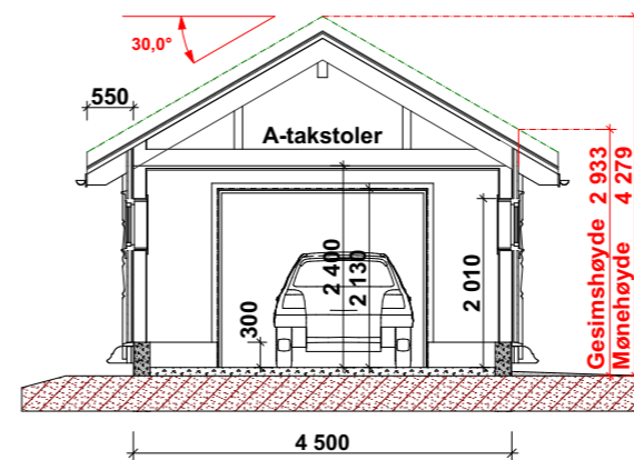
Snitt A-A
