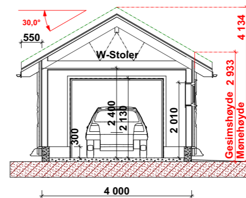
Snitt A-A
