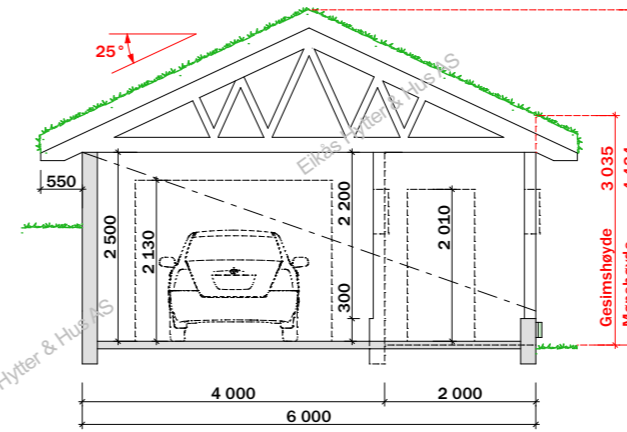
Snitt A-A
