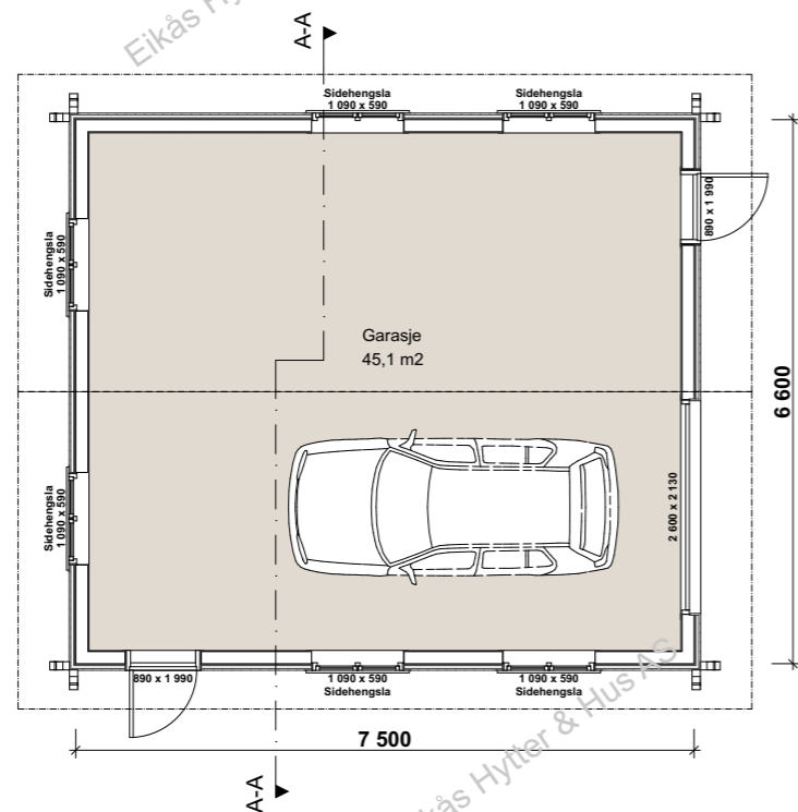
Hovedplan
