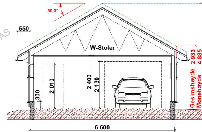
Snitt A-A
