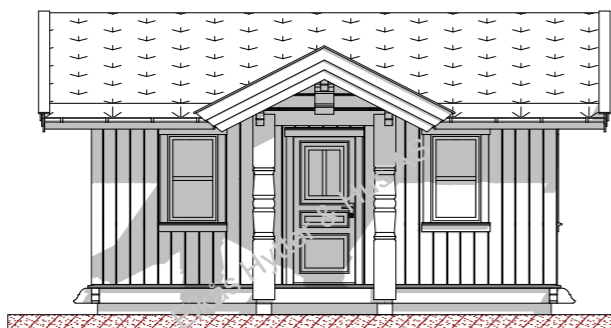
Fasade mot
