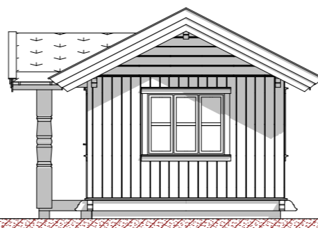
Fasade mot
