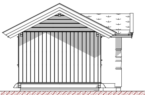
Fasade mot
