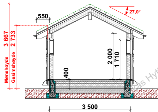
Snitt B-B
