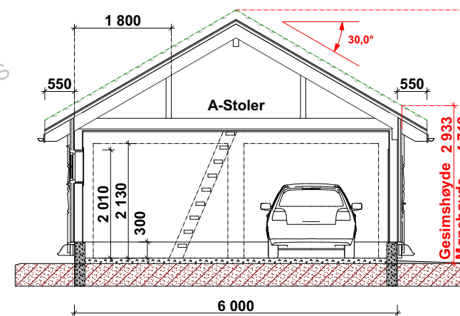
Snitt A-A
