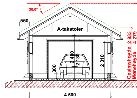
Snitt A-A
