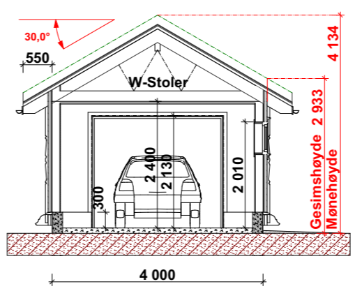
Snitt A-A
