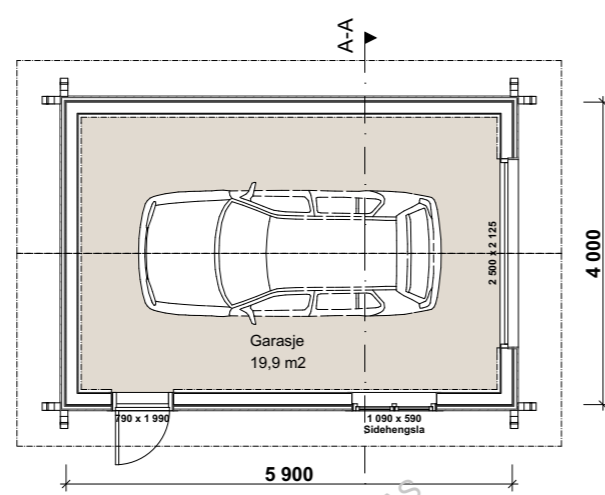
Hovedplan
