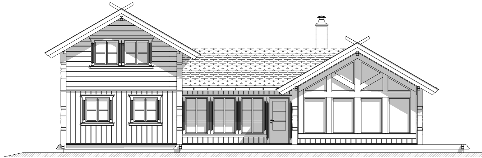
Fasade 1
