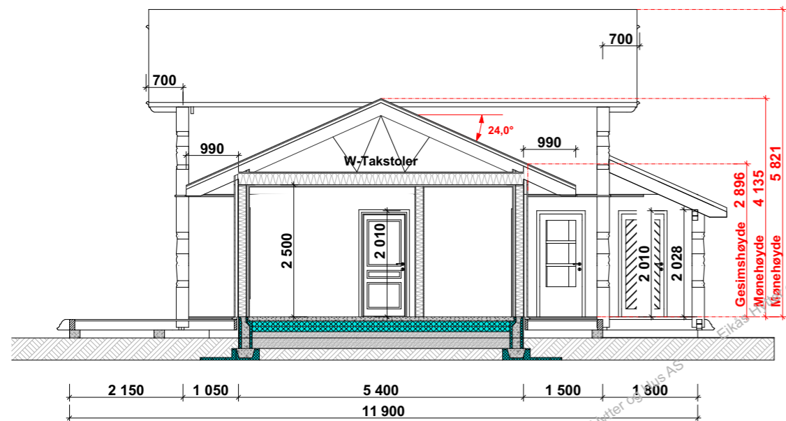
Snitt A-A
