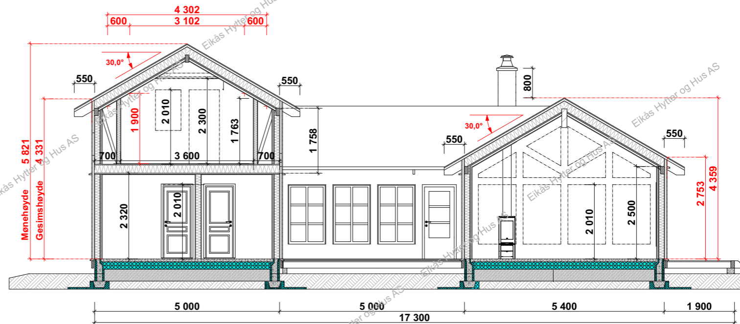
Snitt B-B
