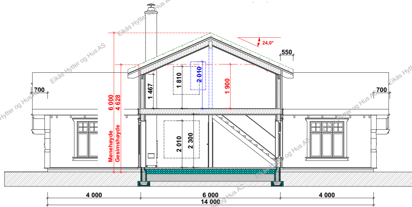
Snitt B-B
