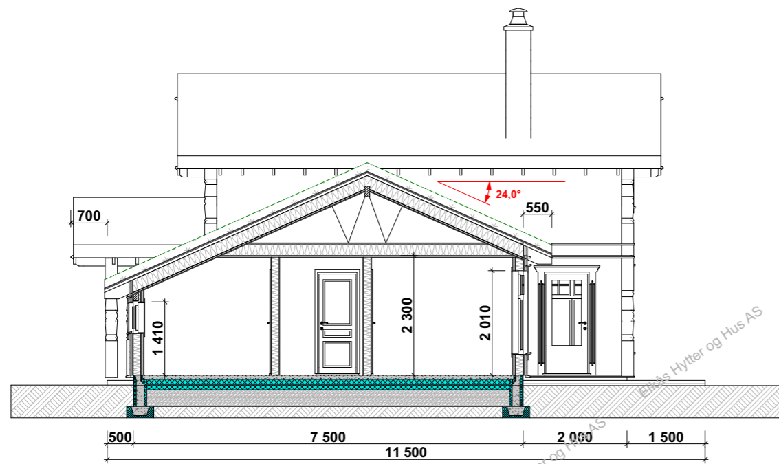
Snitt A-A
