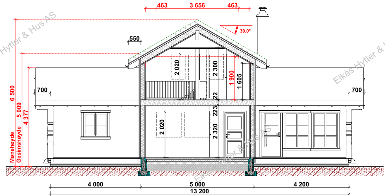
Snitt B-B
