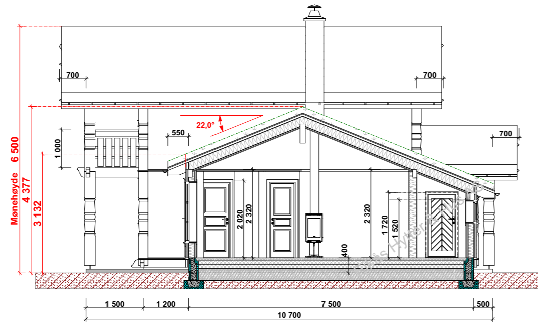
Snitt A-A
