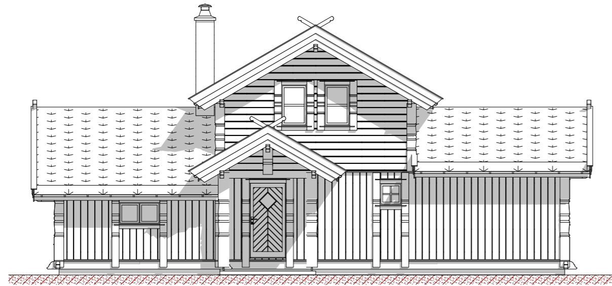
Fasade 1
