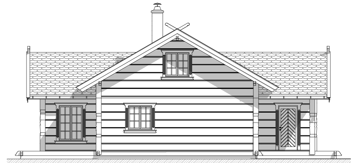
Fasade 4
