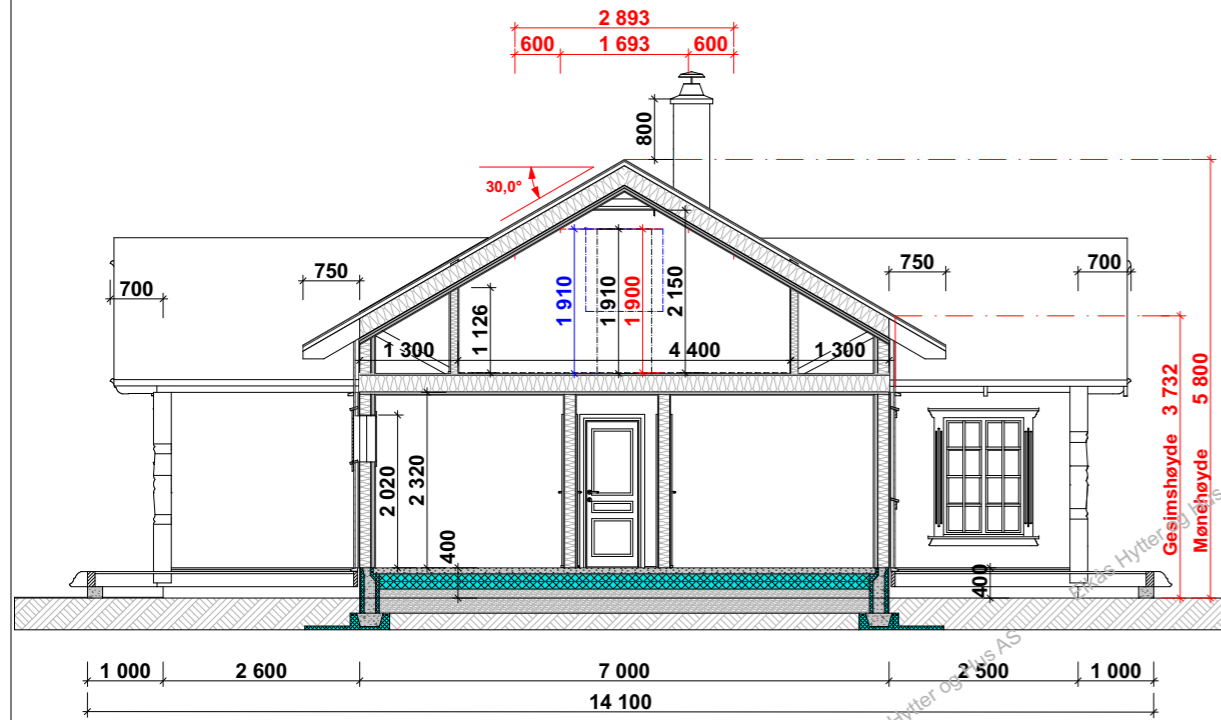
Snitt A-A
