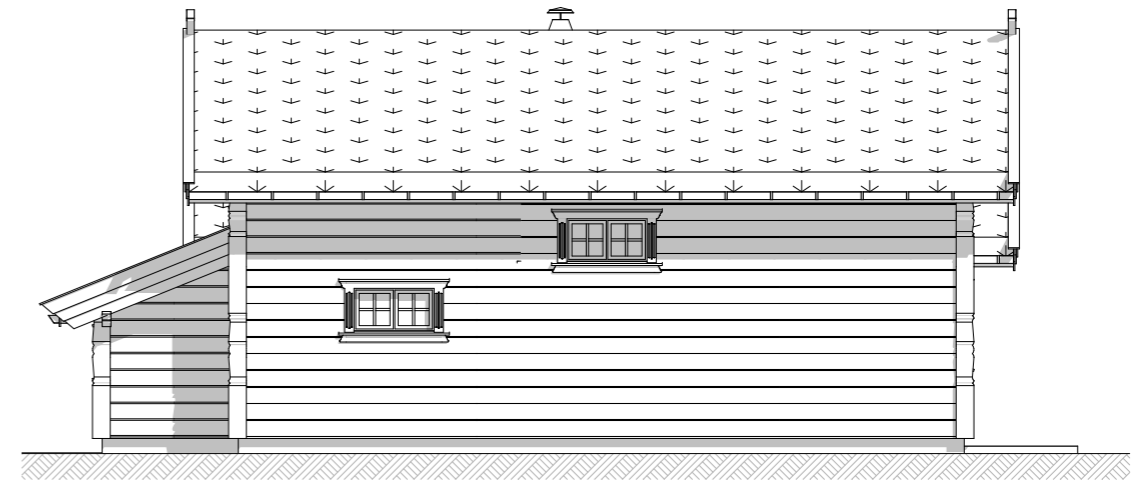
Fasade 2
