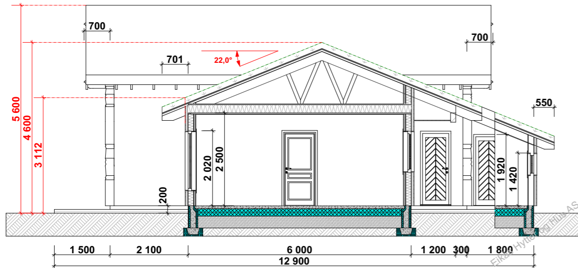
Snitt A-A
