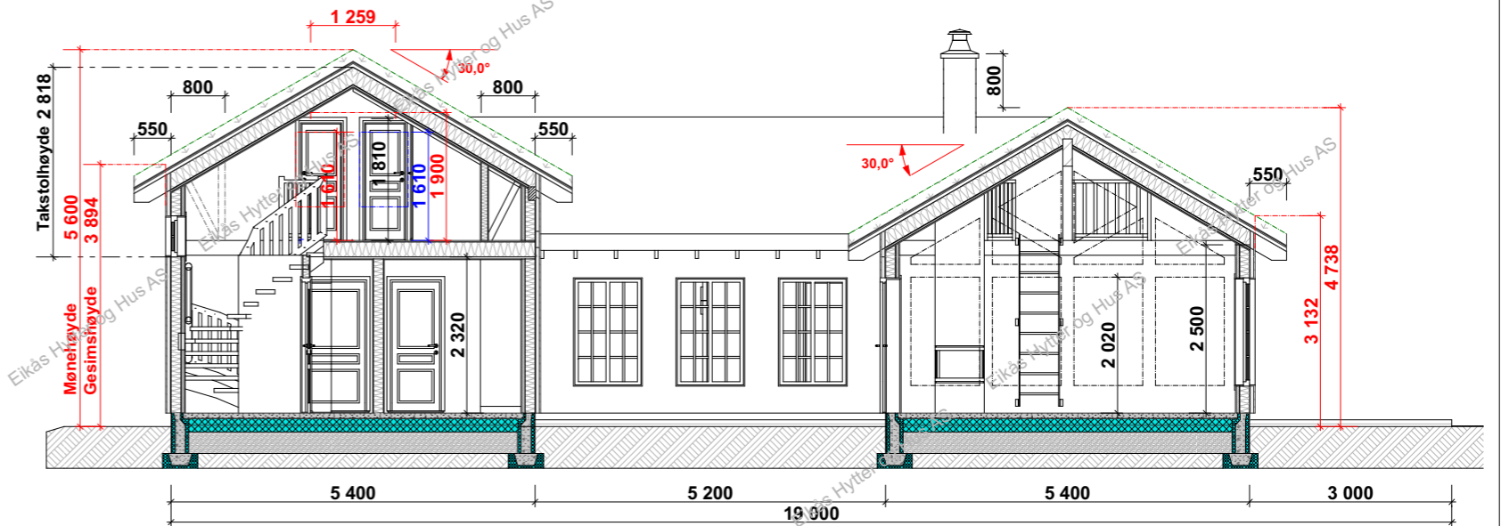
Snitt B-B
