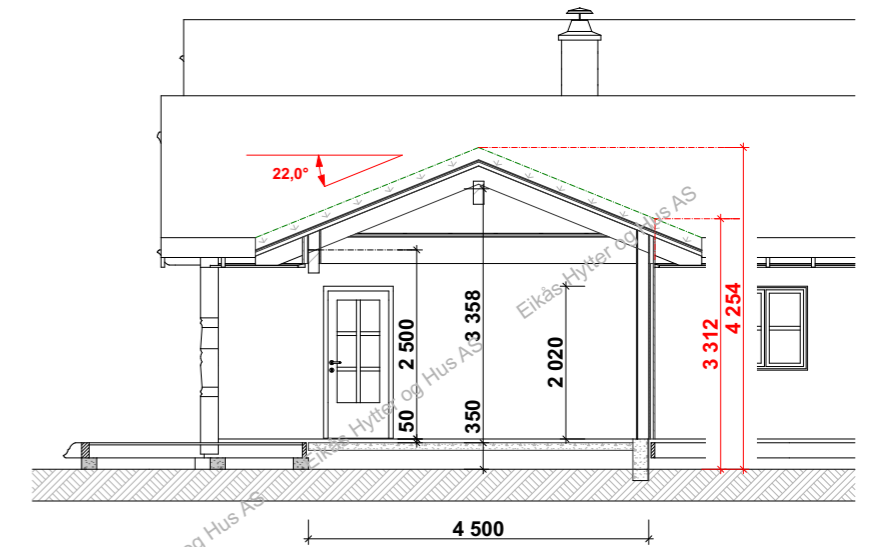
Snitt D-D
