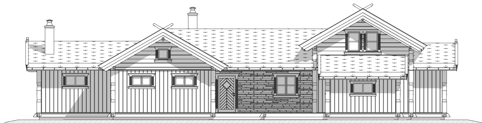
Fasade 3
