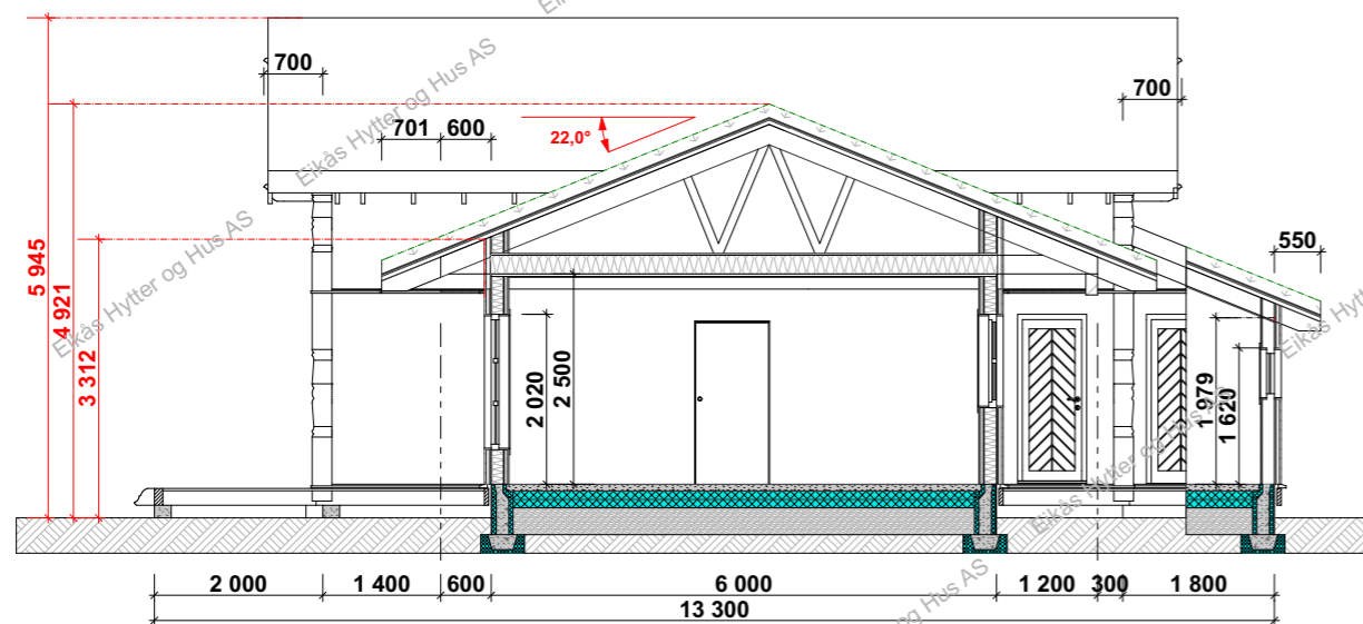
Snitt A-A
