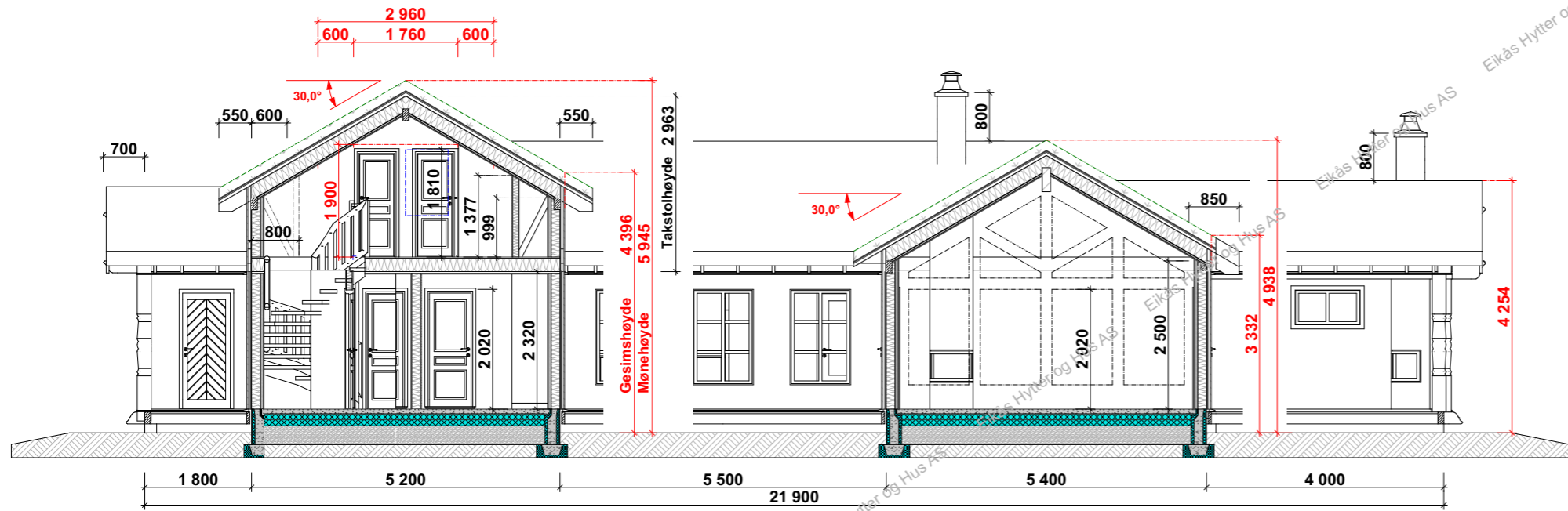
Snitt B-B
