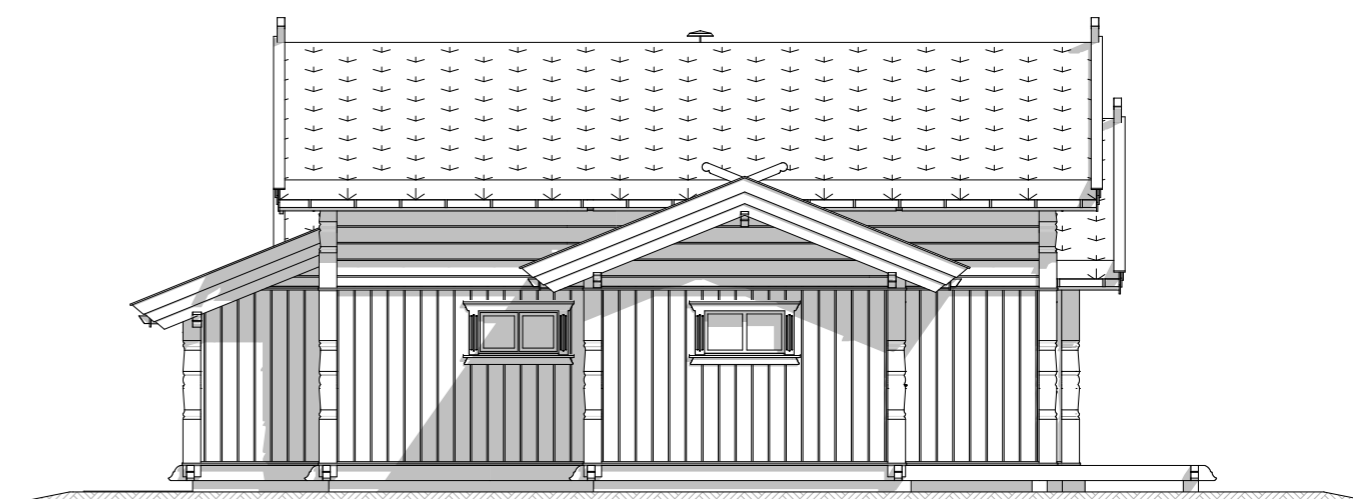
Fasade 4
