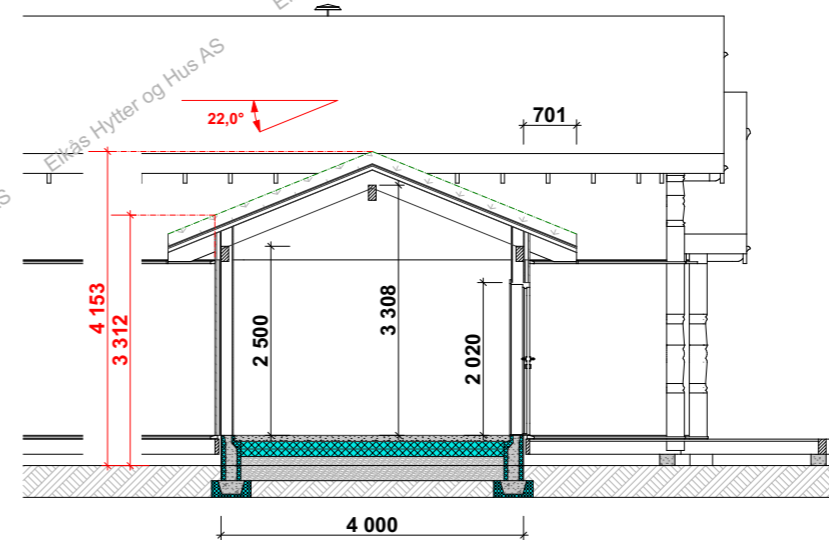
Snitt C-C
