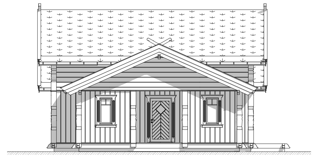
Fasade 4
