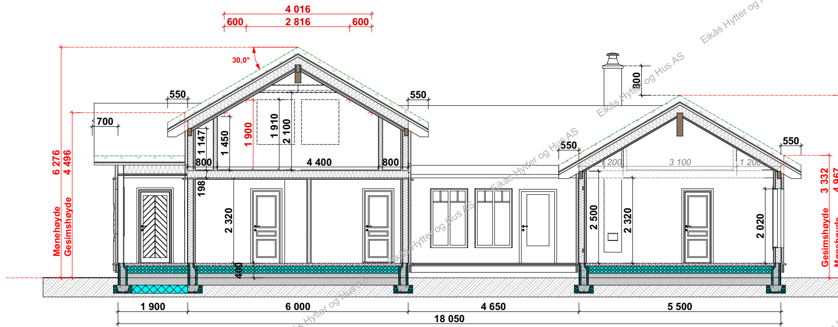
Snitt B-B
