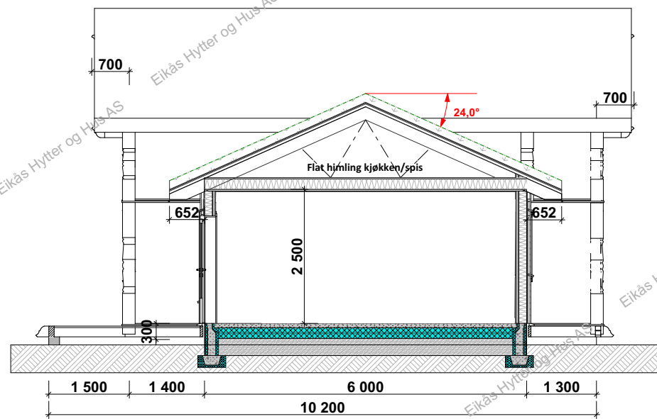
Snitt A-A
