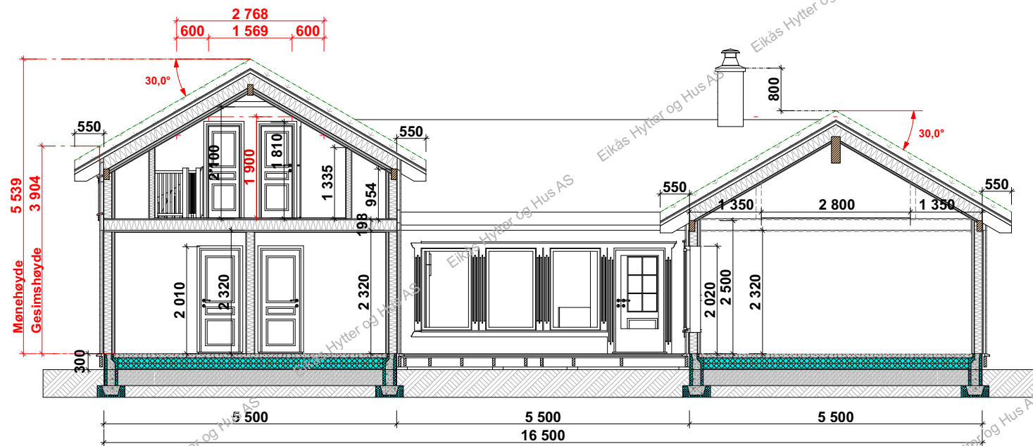
Snitt B-B
