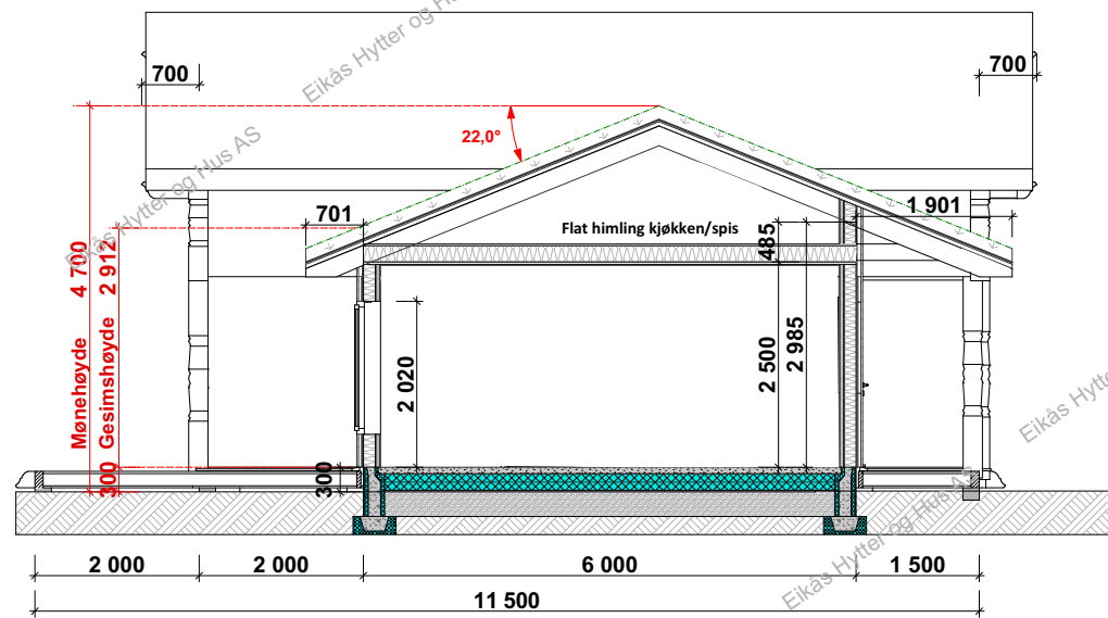
Snitt A-A
