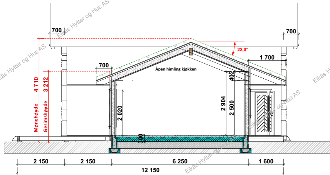
Snitt A-A
