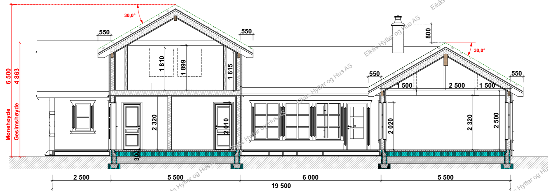
Snitt B-B
