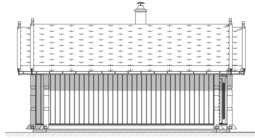
Fasade 2
