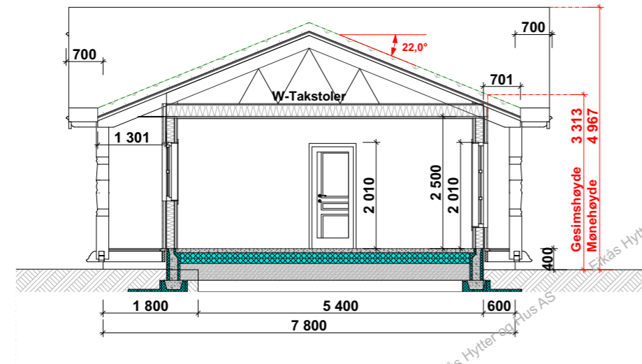
Snitt A-A
