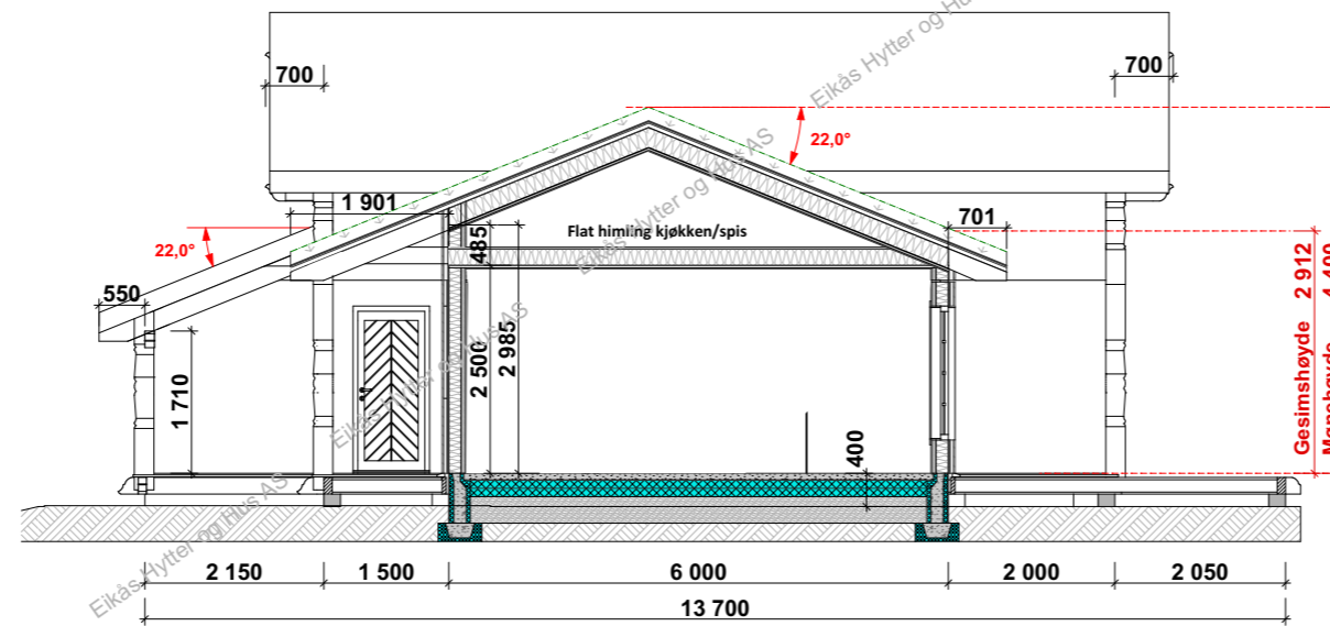
Snitt A-A
