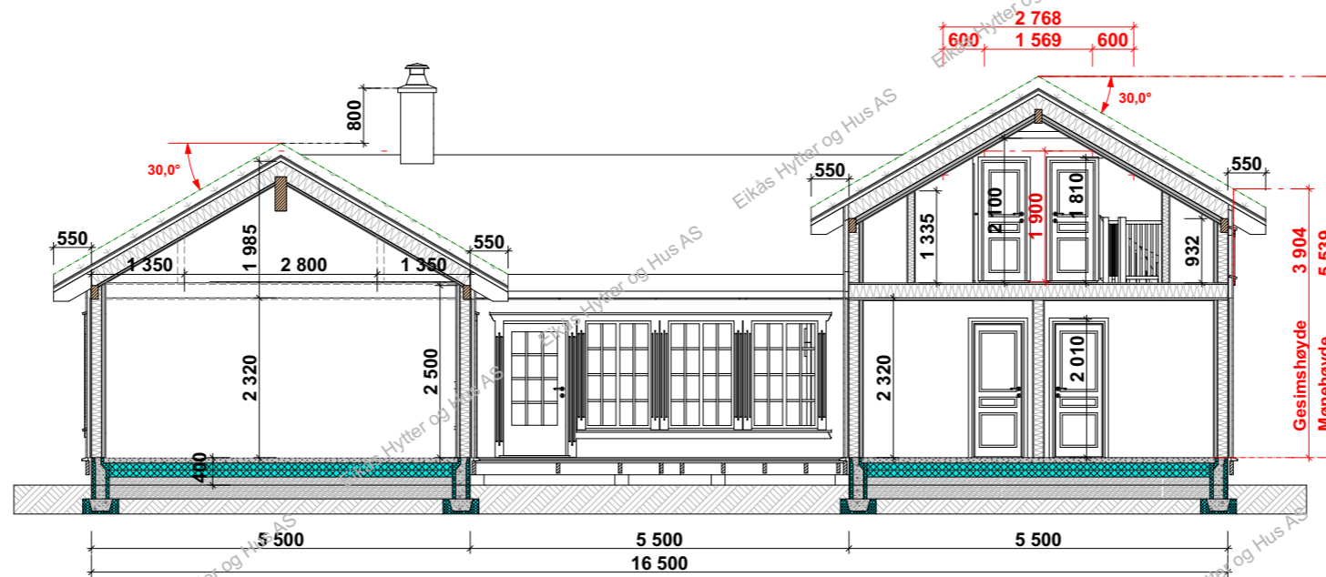
Snitt B-B
