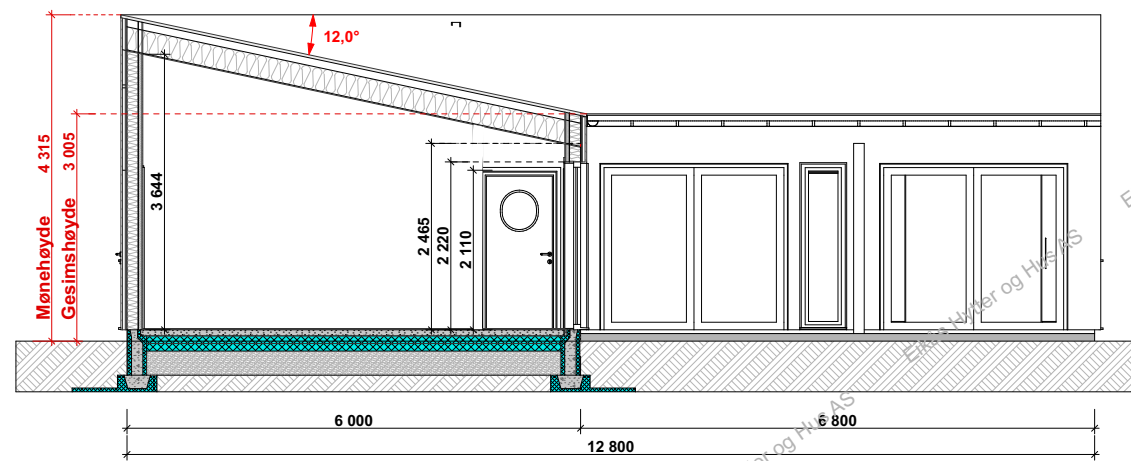
Snitt A-A
