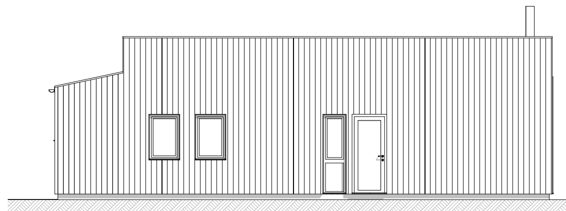
Fasade mot:
