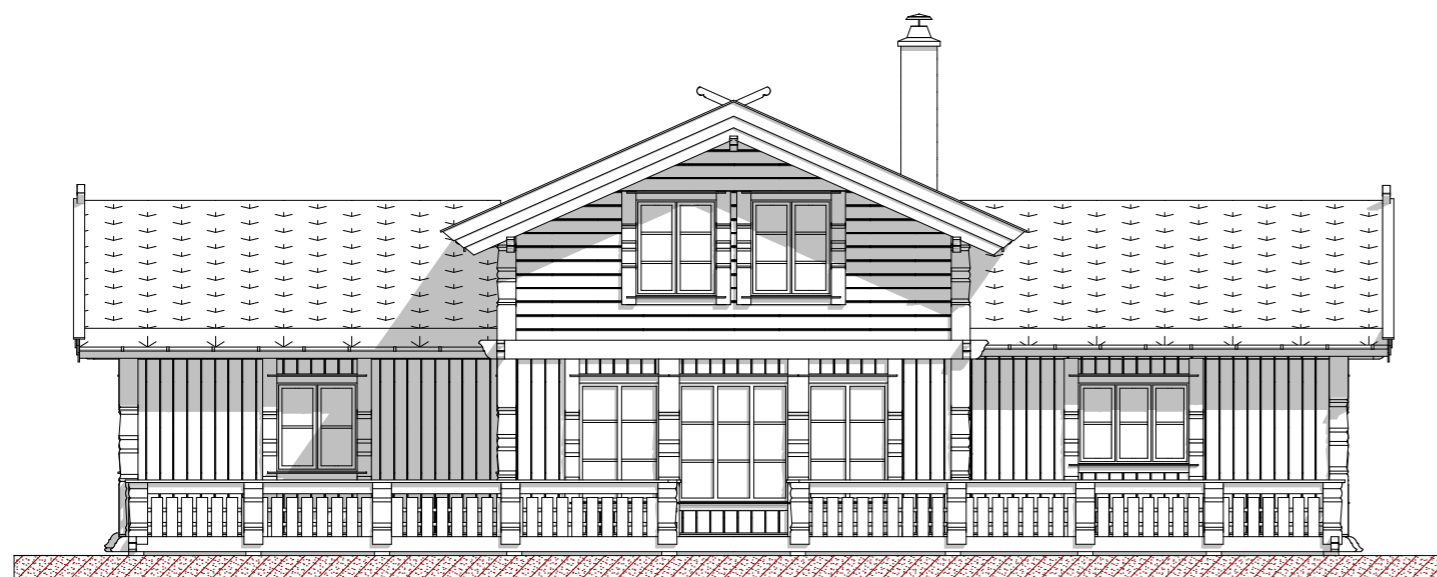
Fasade mot
