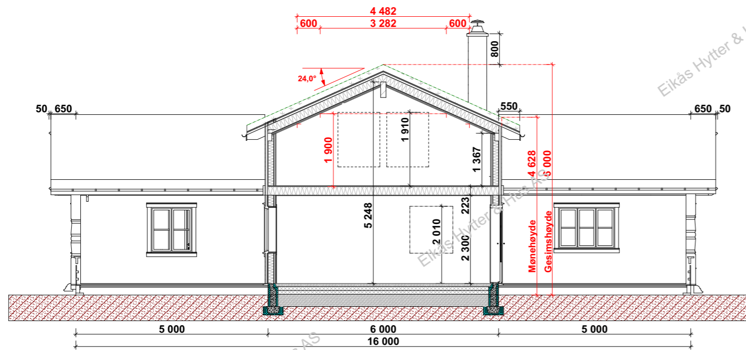
Snitt B-B
