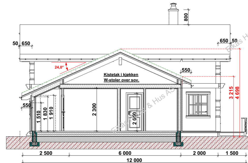
Snitt A-A
