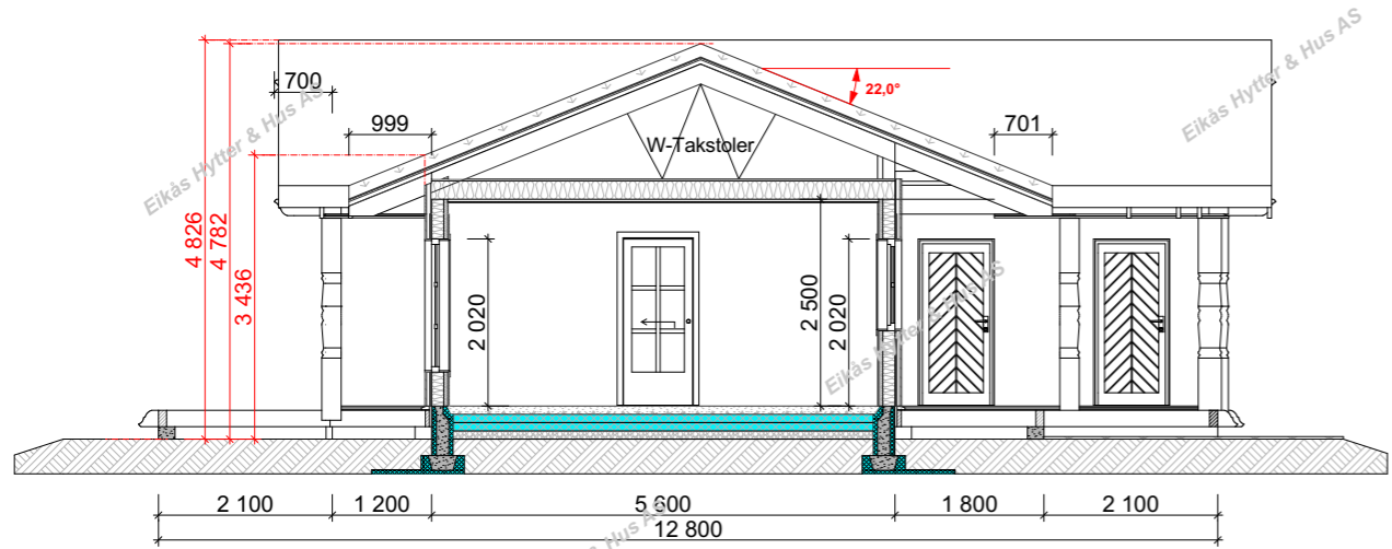
Snitt A-A
