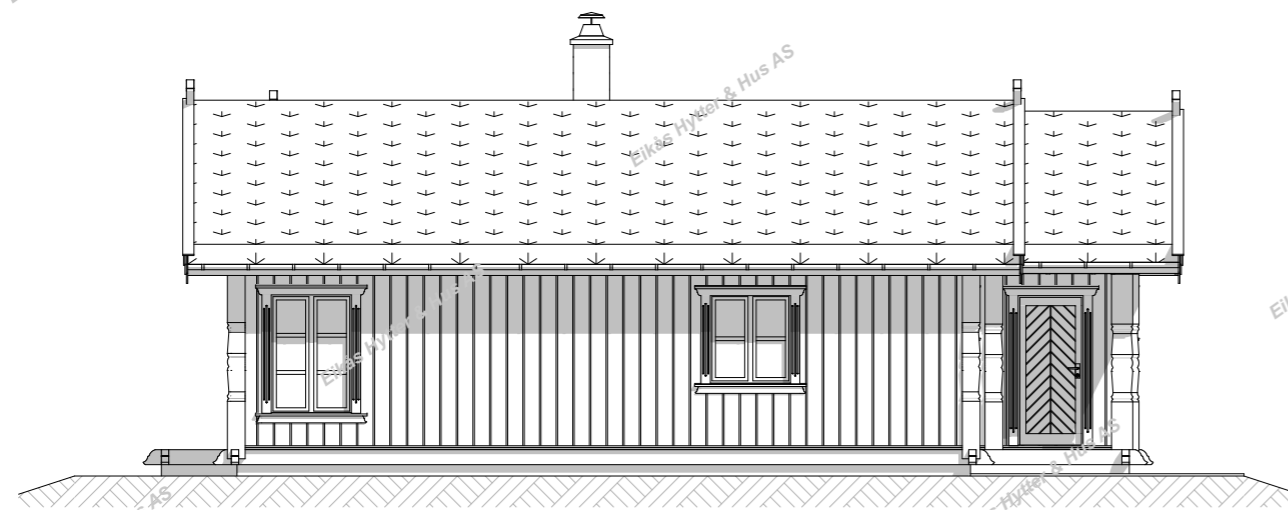
Fasade 2
