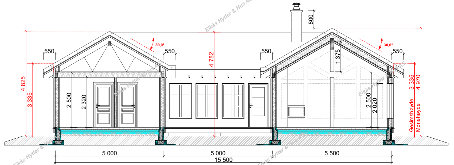
Snitt B-B
