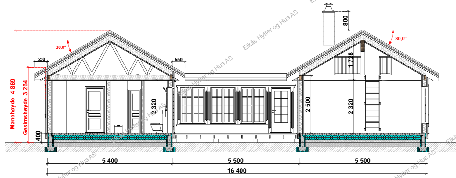
Snitt B-B
