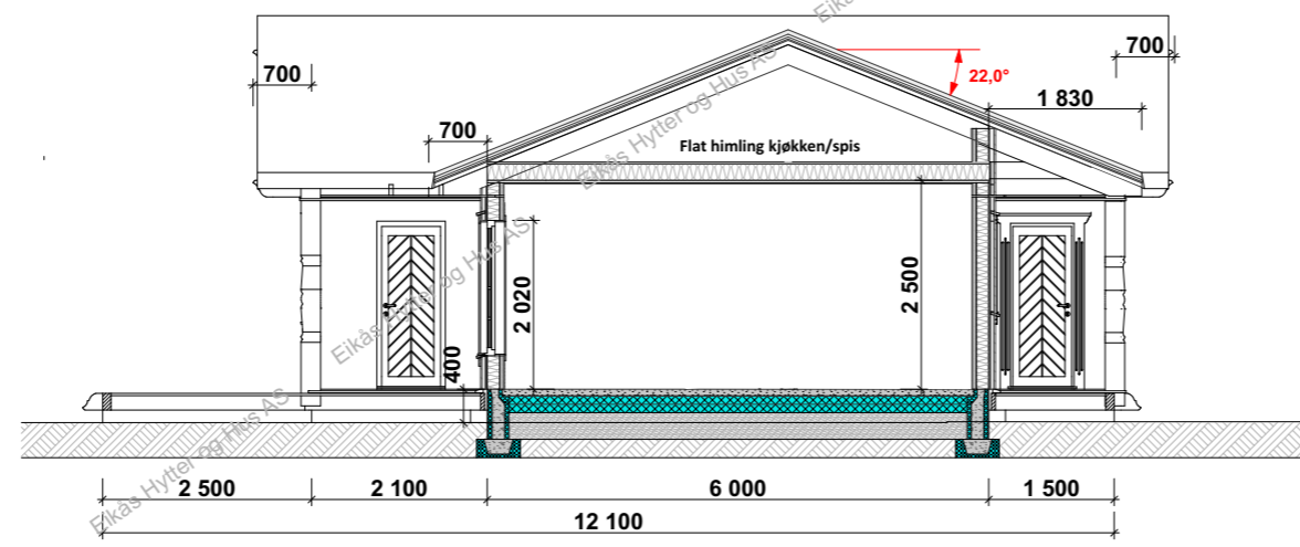
Snitt A-A
