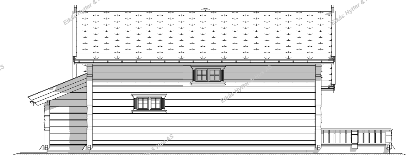
Fasade 4
