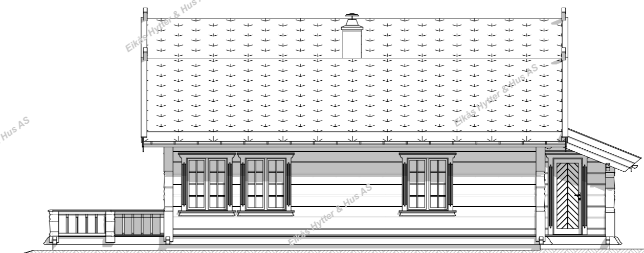
Fasade 2
