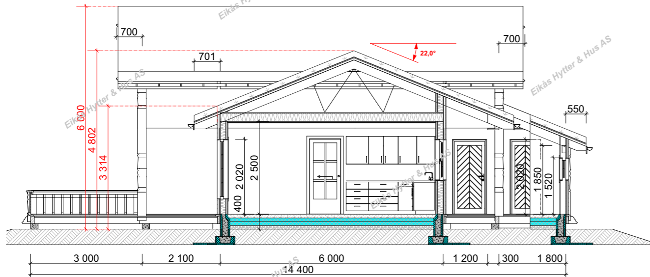
Snitt A-A
