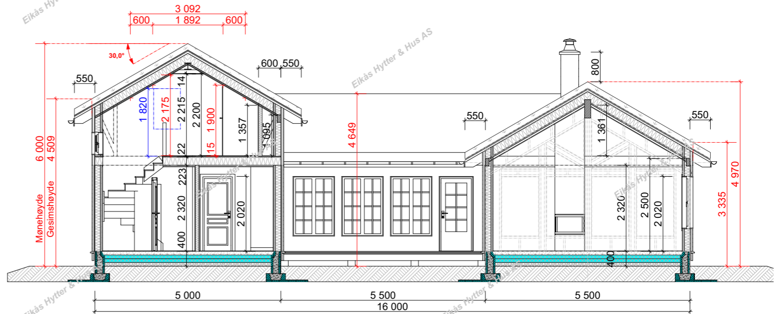
Snitt B-B
