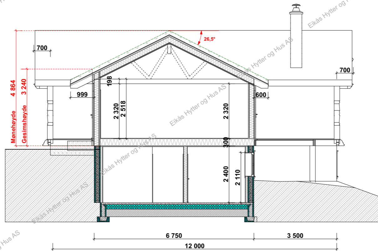
Snitt A-A
