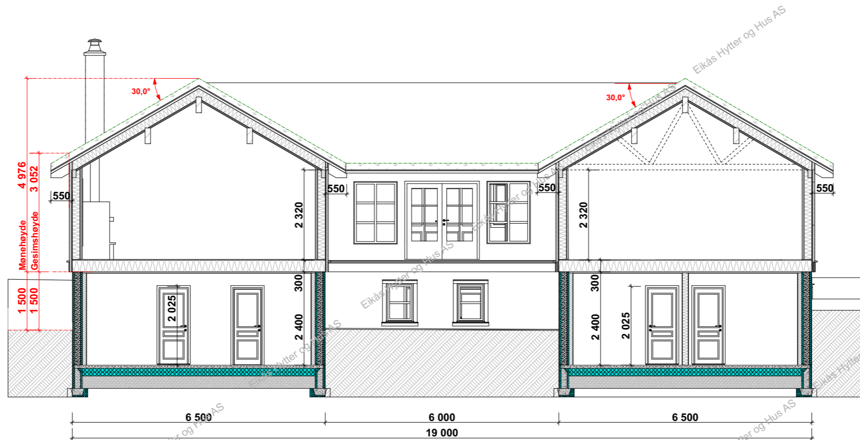
Snitt B-B
