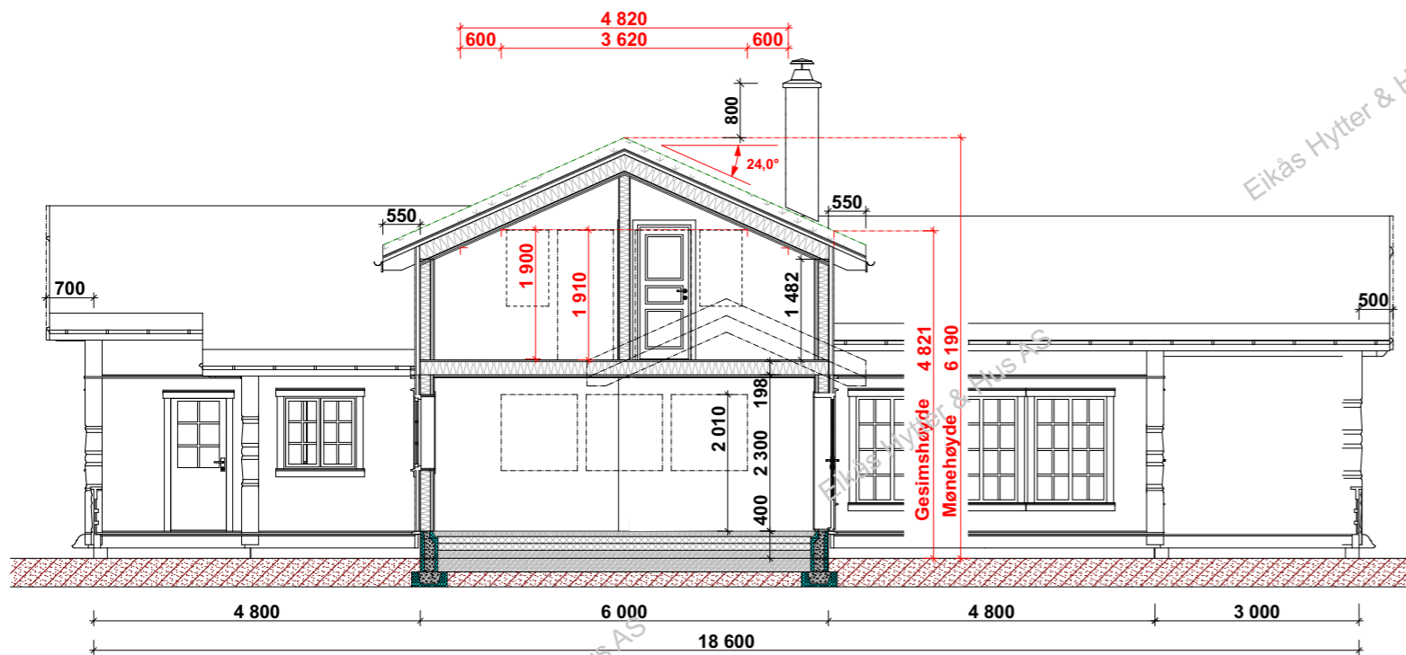
Snitt B-B
