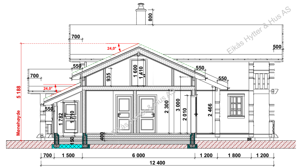
Snitt A-A
