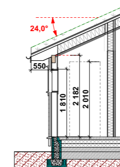
Snitt C-C
