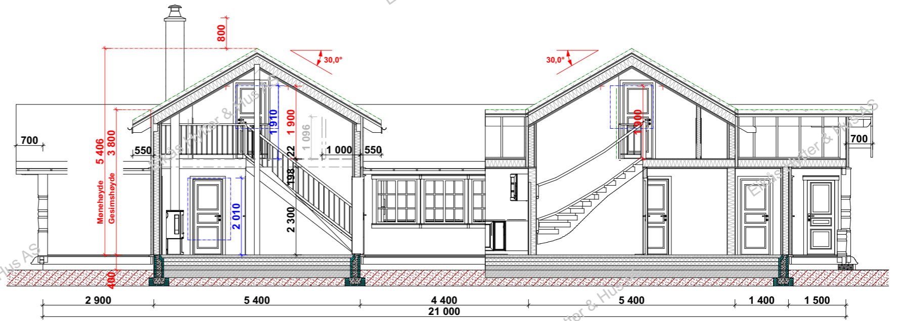
Snitt B-B
