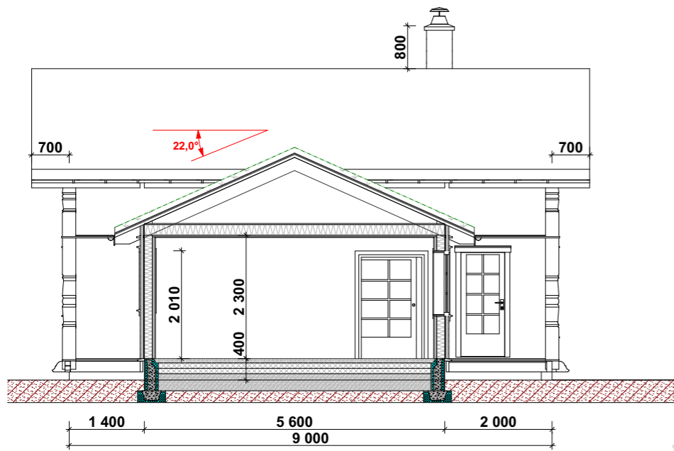
Snitt A-A
