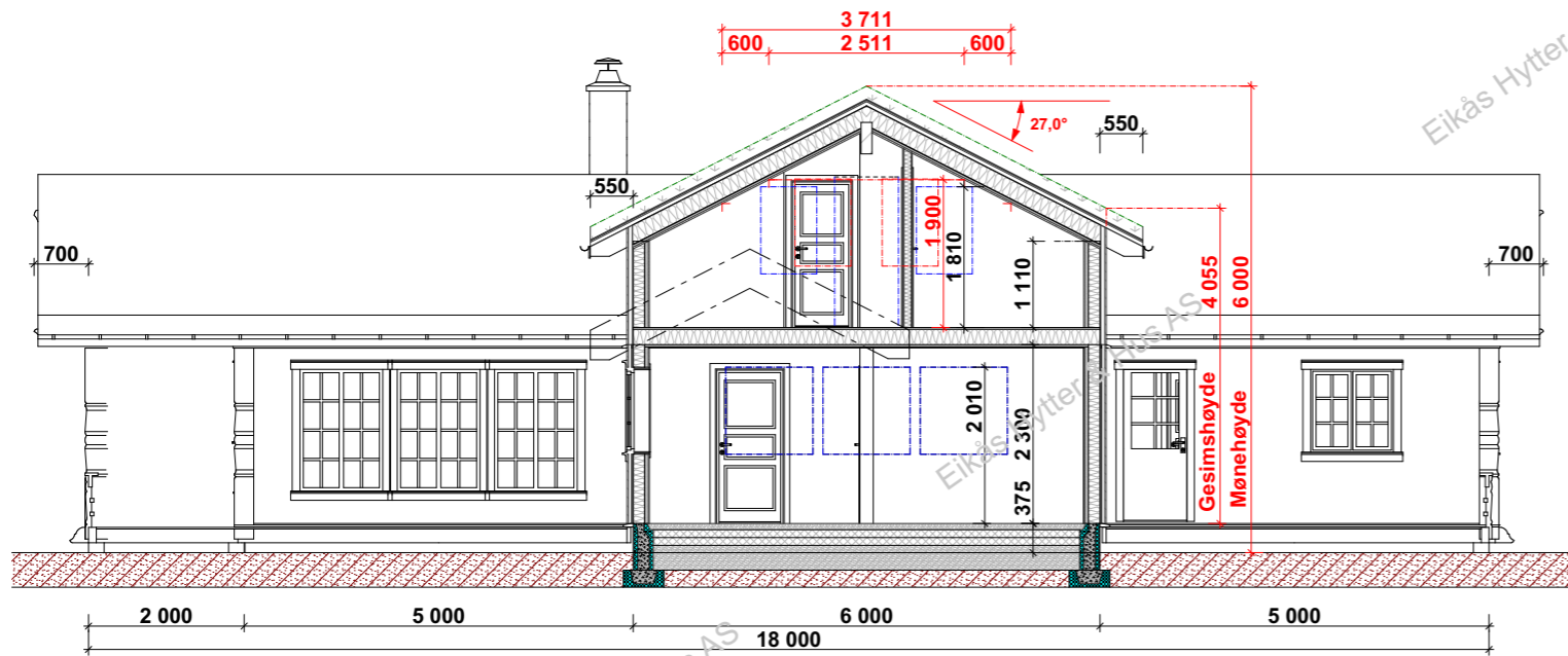
Snitt B-B
