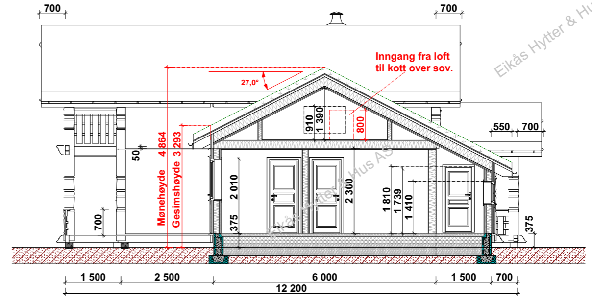
Snitt A-A
