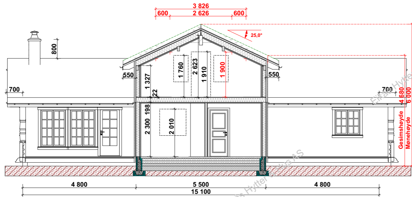
Snitt B-B
