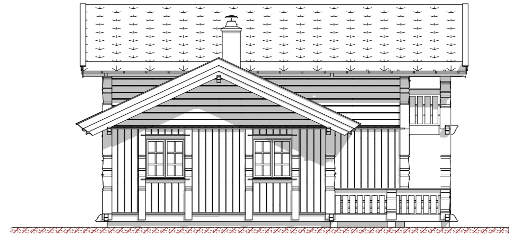
Fasade mot
