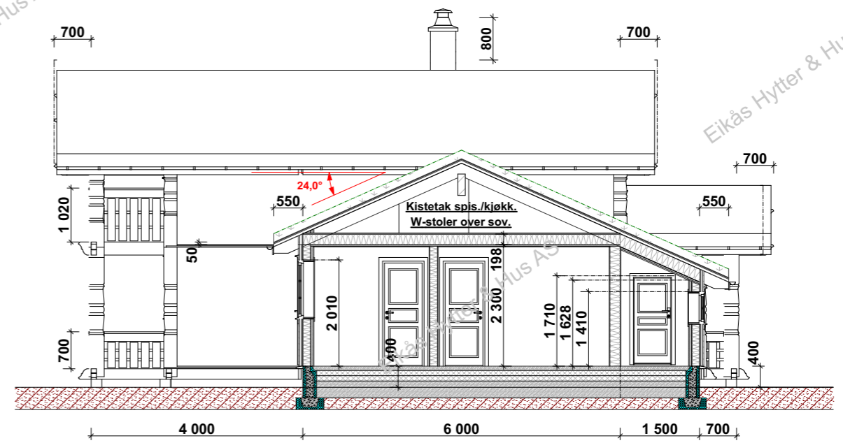
Snitt A-A
