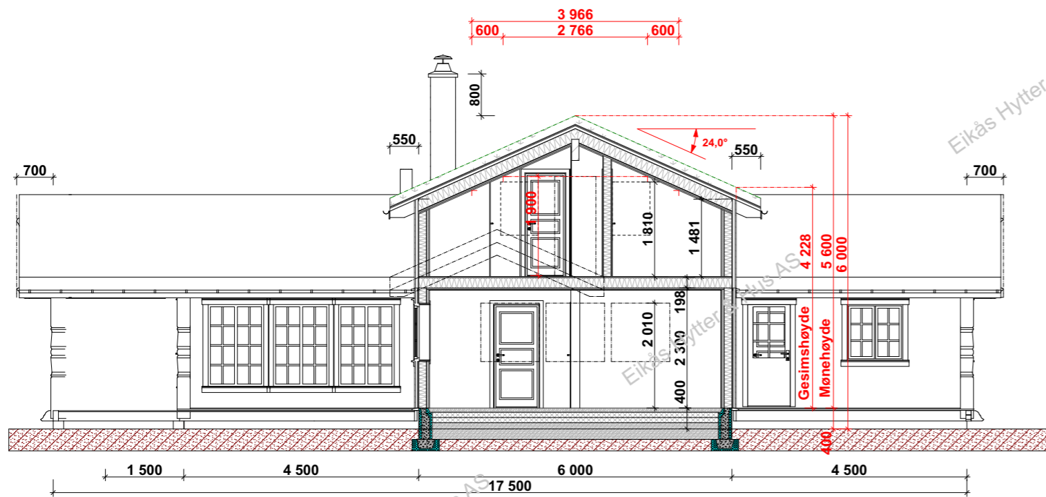
Snitt B-B
