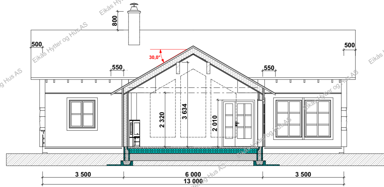
Snitt B-B
