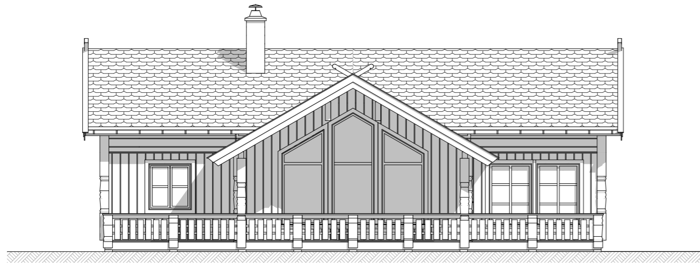
Fasade mot:
