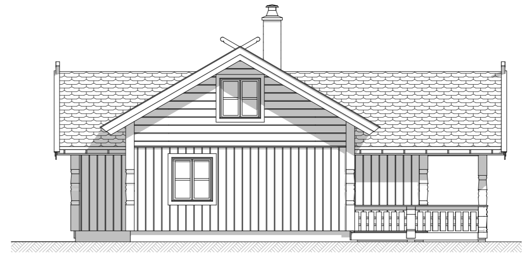
Fasade mot:
