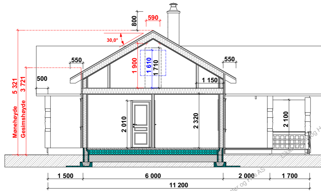
Snitt A-A
