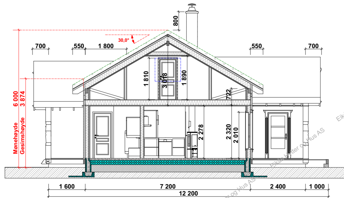
Snitt A-A
