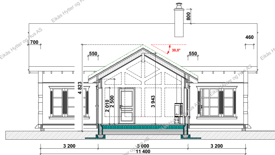
Snitt B-B
