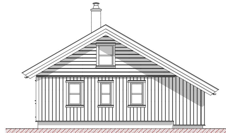
Fasade mot
