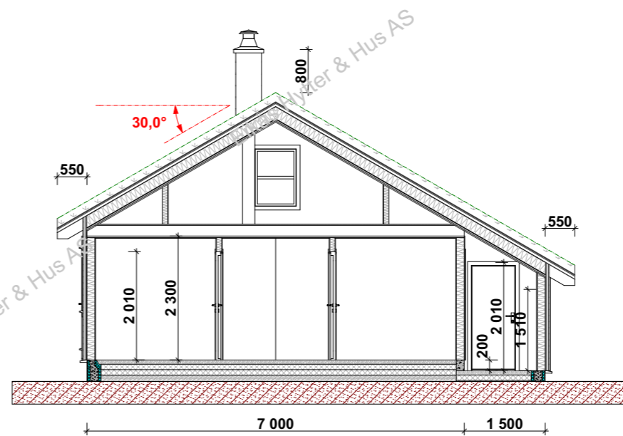
Snitt B-B
