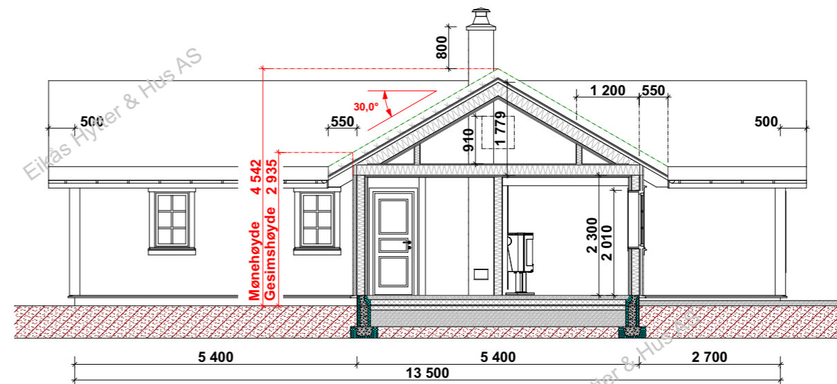
Snitt A-A
