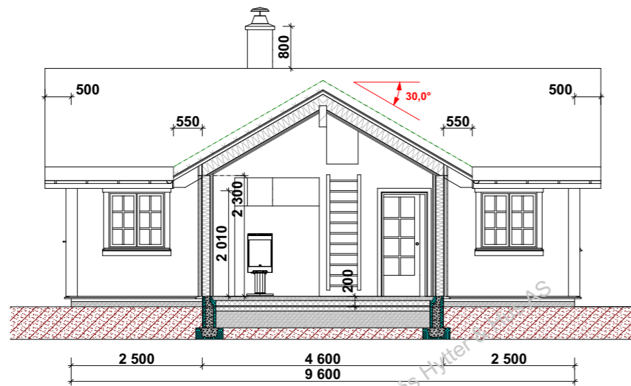
Snitt B-B
