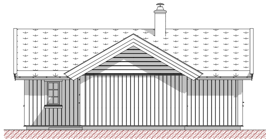
Fasade mot
