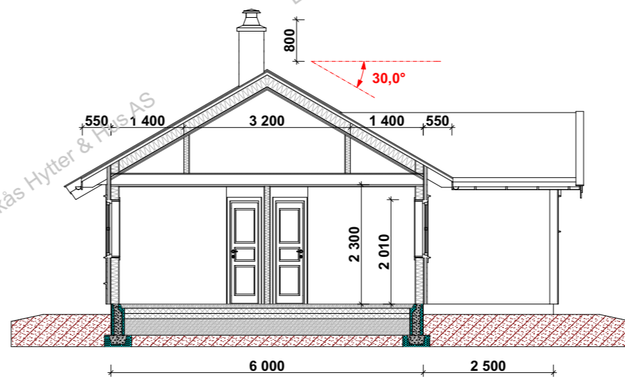
Snitt B-B
