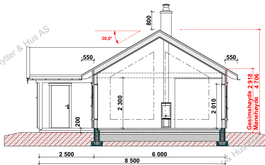
Snitt A-A
