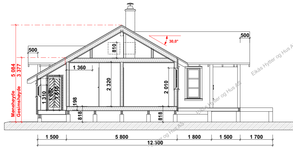
Snitt A-A
