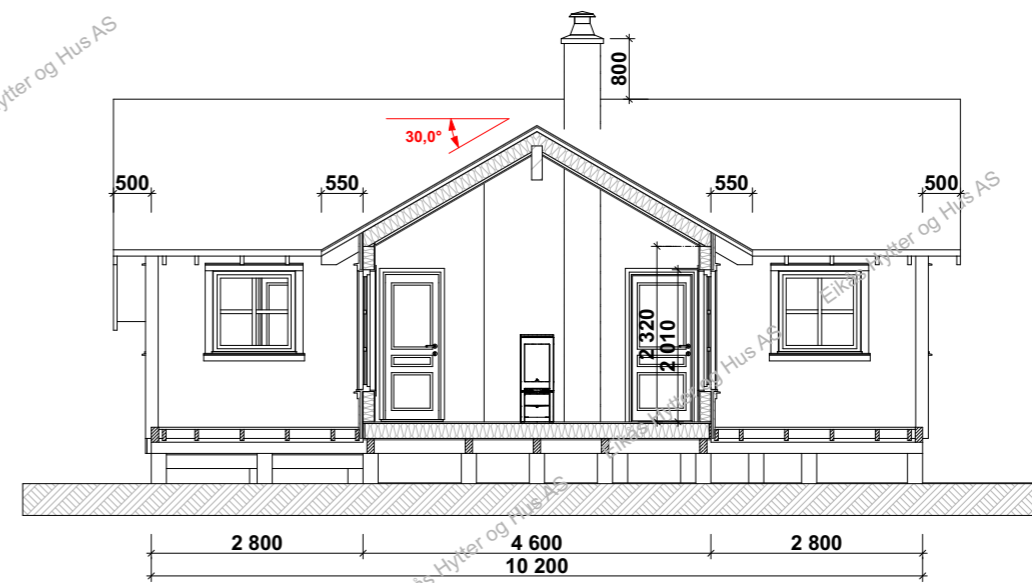
Snitt B-B
