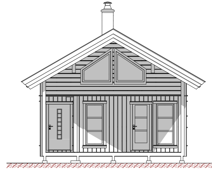
Fasade mot
