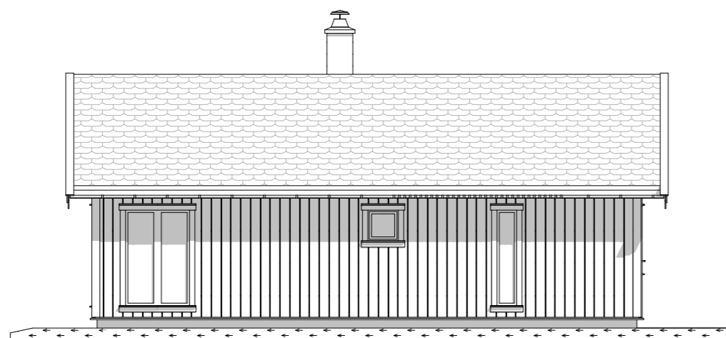
Fasade mot
