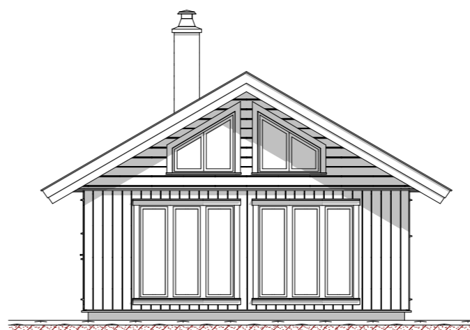
Fasade mot
