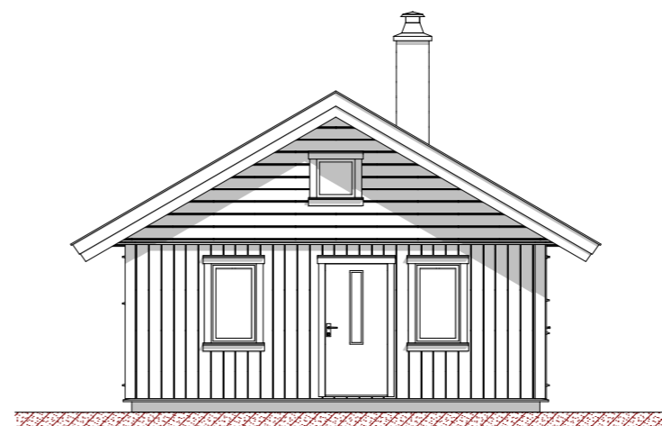
Fasade mot
