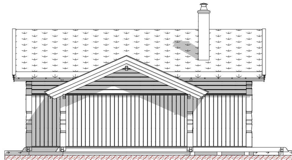
Fasade mot
