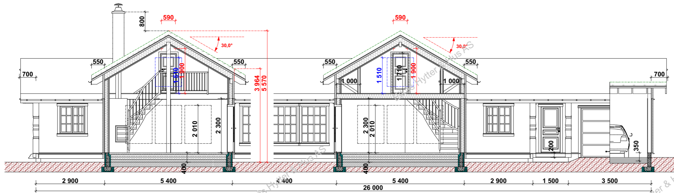
Snitt B-B
