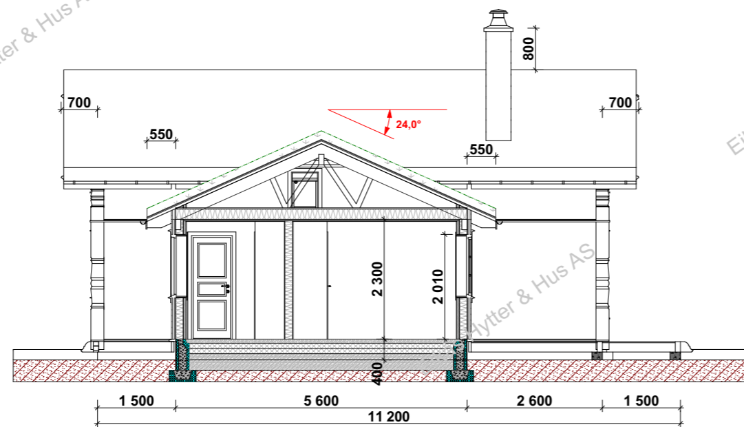
Snitt A-A
