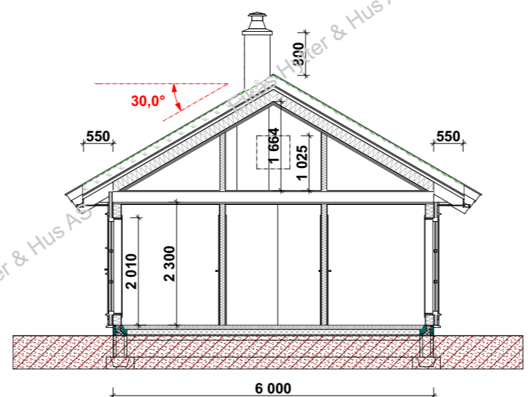
Snitt B-B
