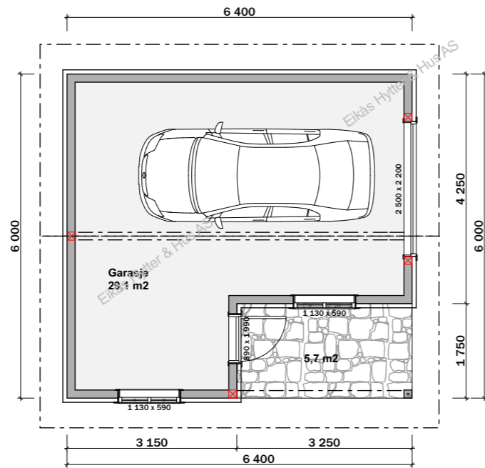
Hovedplan
