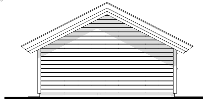
Fasade mot
